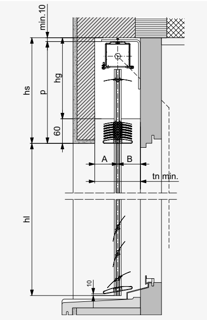
Secciones horizontales
