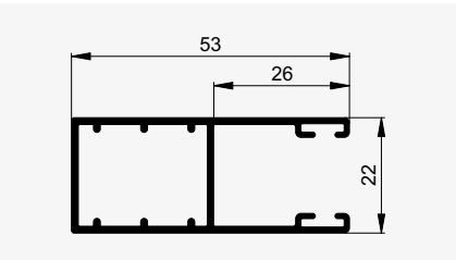
Rieles guía (standard)
