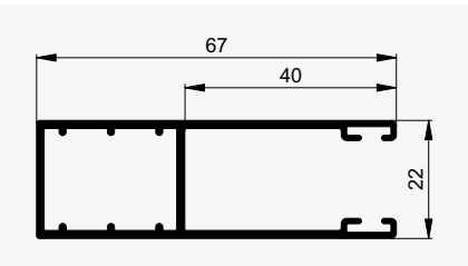
Guía empotrada (opción)
