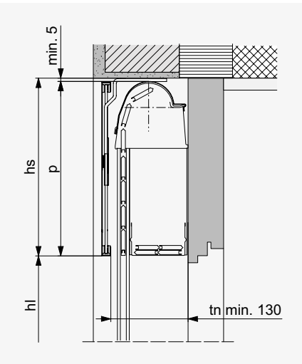
Sección vertical: ejemplo tapa
