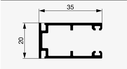
GUÍAS LATERALES
